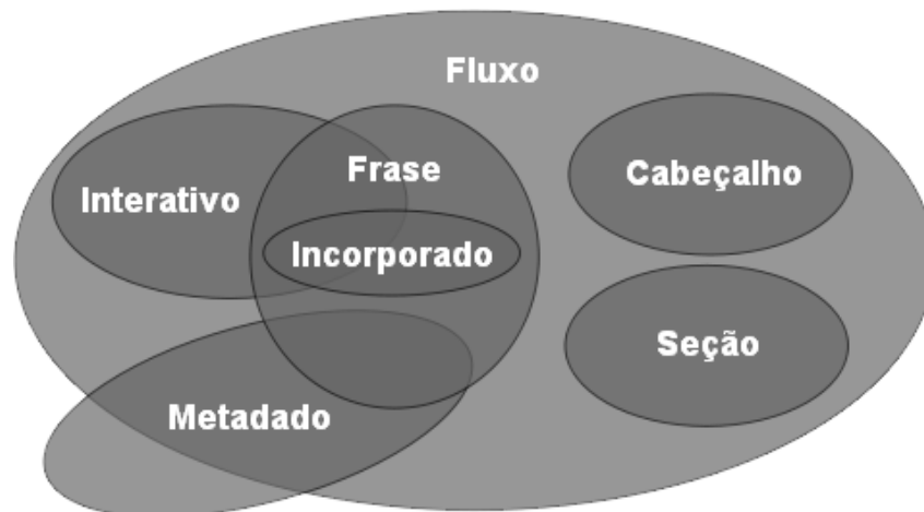
Figura 2.1 – Modelo de conteúdo.
