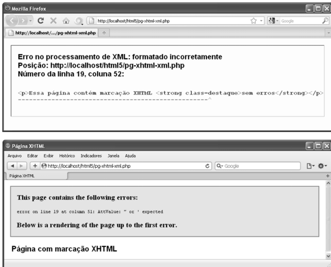
Figura 1.1 – Erro em documento XHTML em navegador standard.
