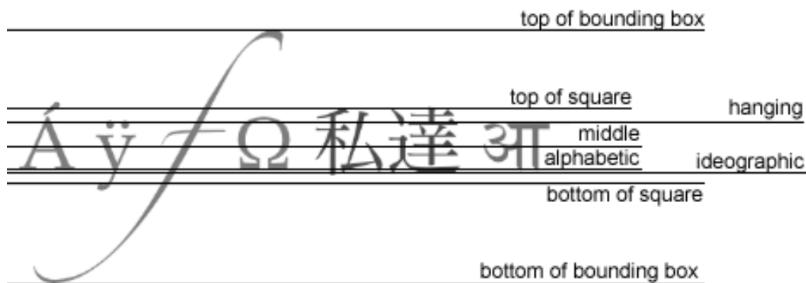
Figura 4.5 – Linhas de base para textos.
