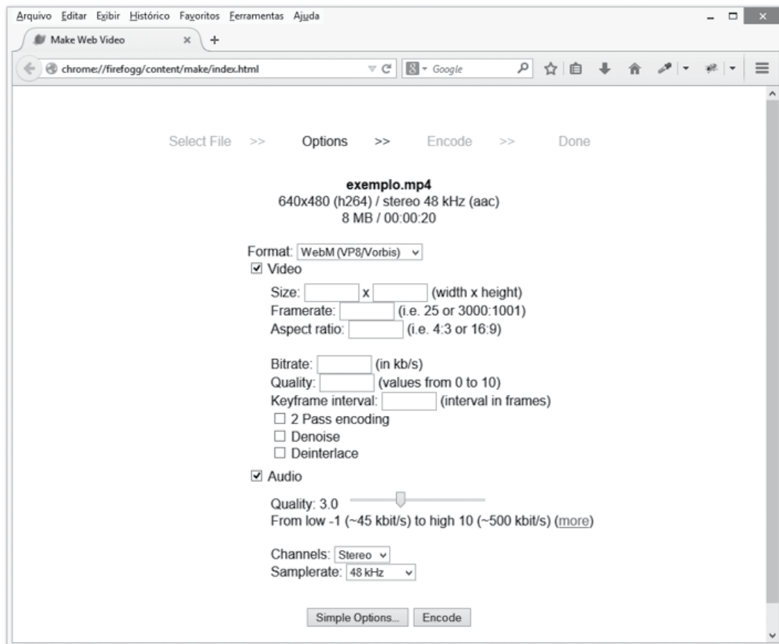
Figura 3.14 – Menu de configurações avançadas.
