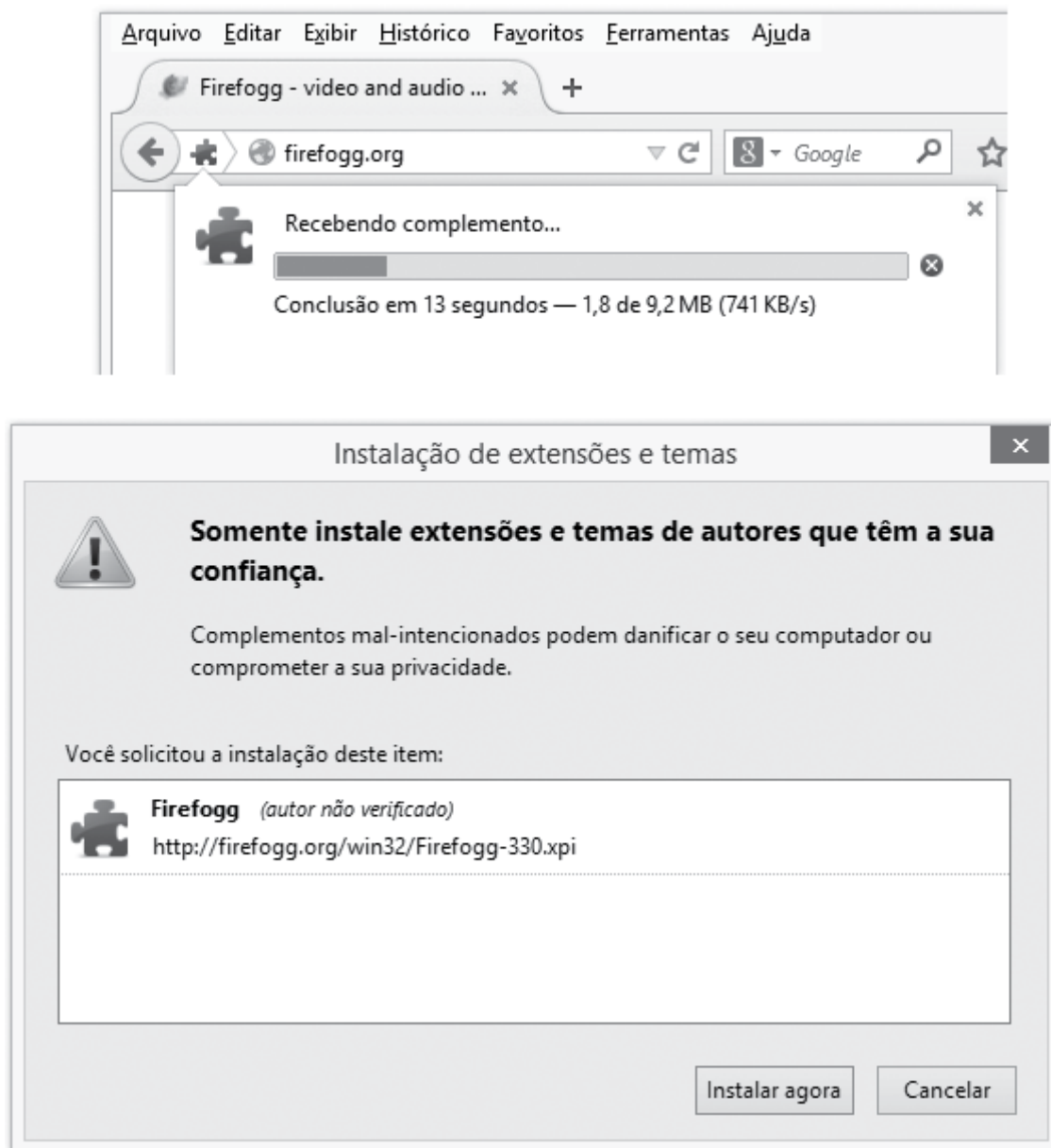
Figura 3.5 – Iniciar instalação.
