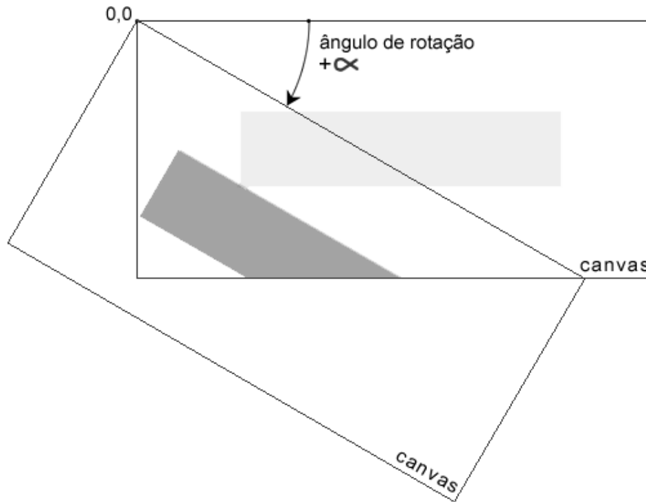
Figura 4.3 – Mecanismo para rotate() .
